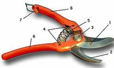
Onderdelen van een snoeischaar. 1 groot blad, 2 klein blad, 3 draaipunt, 4 veerbevestiging, 5 veer, 6 handvat, 7 buitenbeugel om de schaar gesloten te houden.
